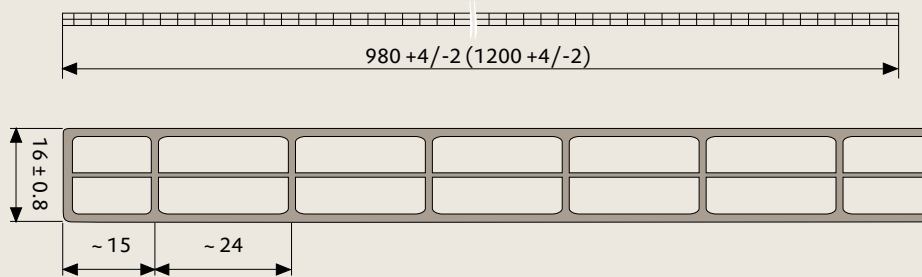
Querschnitt der PLEXIGLAS® Resist S3P 16 (Maße in mm)
