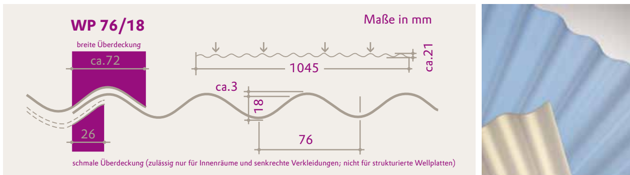
Querschnitt der PLEXIGLAS HEATSTOP® Cool Blue WP 76/18 (Maße in mm)
