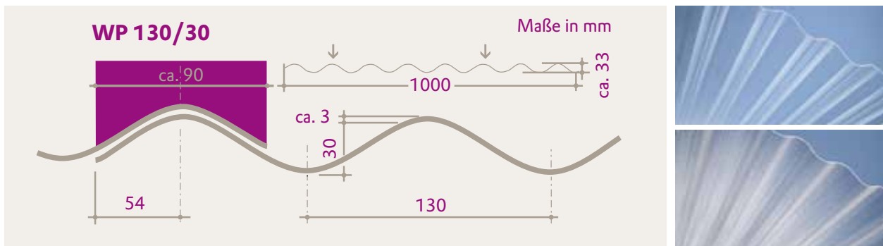
Querschnitt der PLEXIGLAS RESIST® WP 130/30 (Maße in mm)
