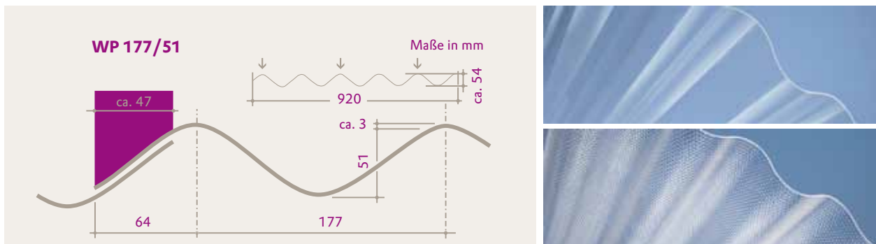
Querschnitt der PLEXIGLAS RESIST® WP 177/51 (Maße in mm)
